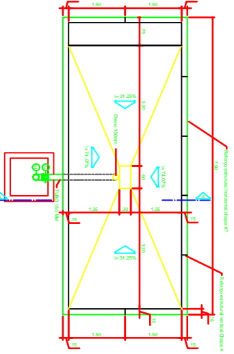
Det. 06 - Detalhe do fundo do decantador. Escala 1:25
